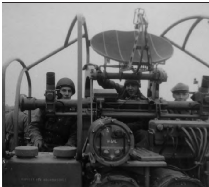
Siktet bemannat av fr.v. menige Halldin, Hedström och Liljegren. Texten längst ner t.v. på siktet lyder "Kopplat till målangivare".
